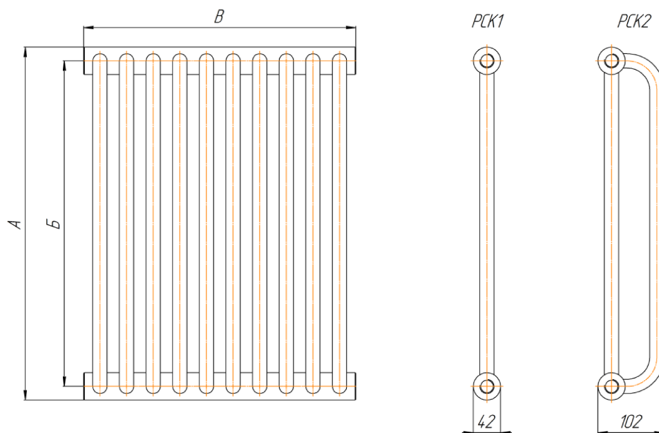
Рис. 1.2 Модификации радиаторов «РСК».
