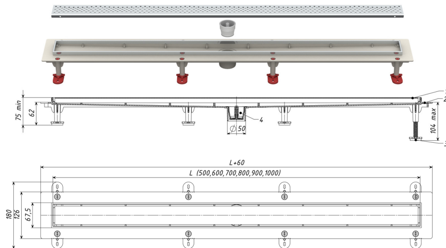
Рис. 1 – Габаритные размеры
