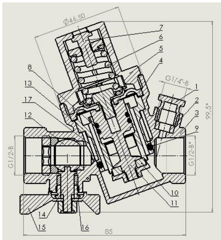
Рисунок 1 – Общий вид и габаритные размеры
