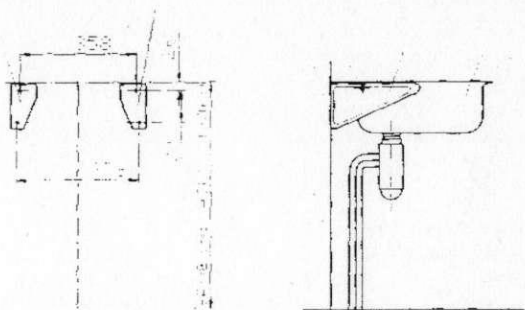
1- мойка ; 2 - кронштейн левый; 3 - кронштейн правый; 4 - болт М6х25 ГОСТ 7801; 5 - гайка М6 ГОСТ 5915; 6 - шайба 6 ГОСТ 11371
